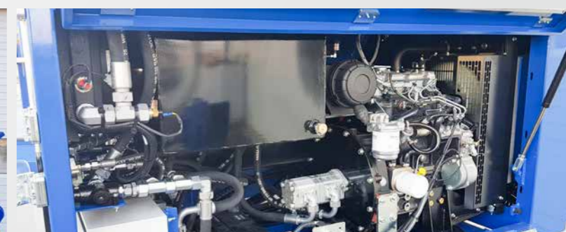
Moteur diesel 25 kW avec une très basse consommation 8 de carburant
